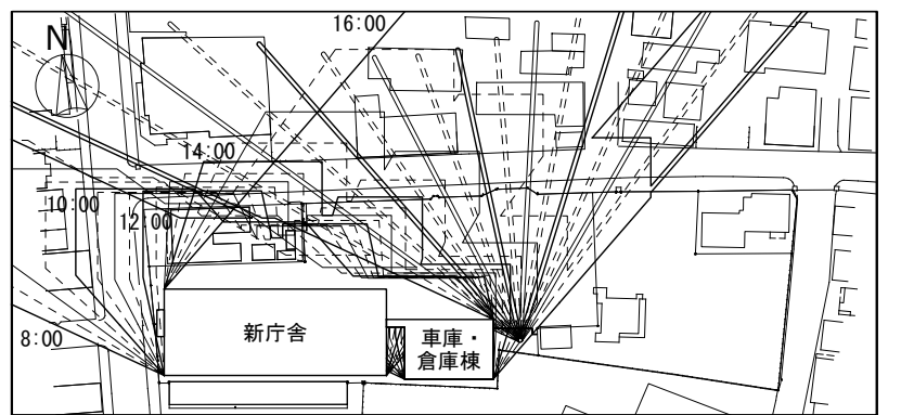
時間別日影図 S=1/2,000
