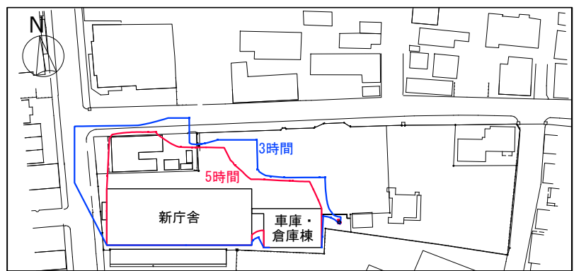
等時間日影図 S=1/2,000
