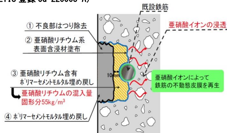
リハビリ断面修復工法 概念図
