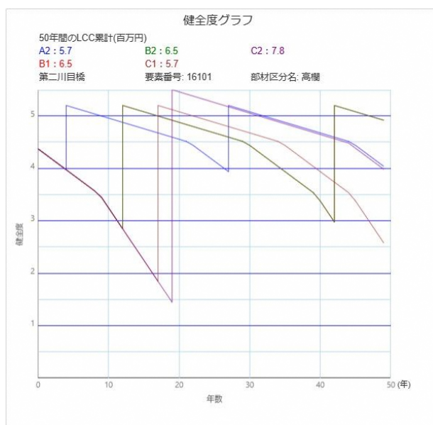
図 7-7 健全度グラフ例
